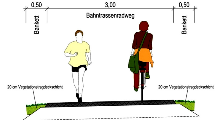
Ausbauquerschnitt
